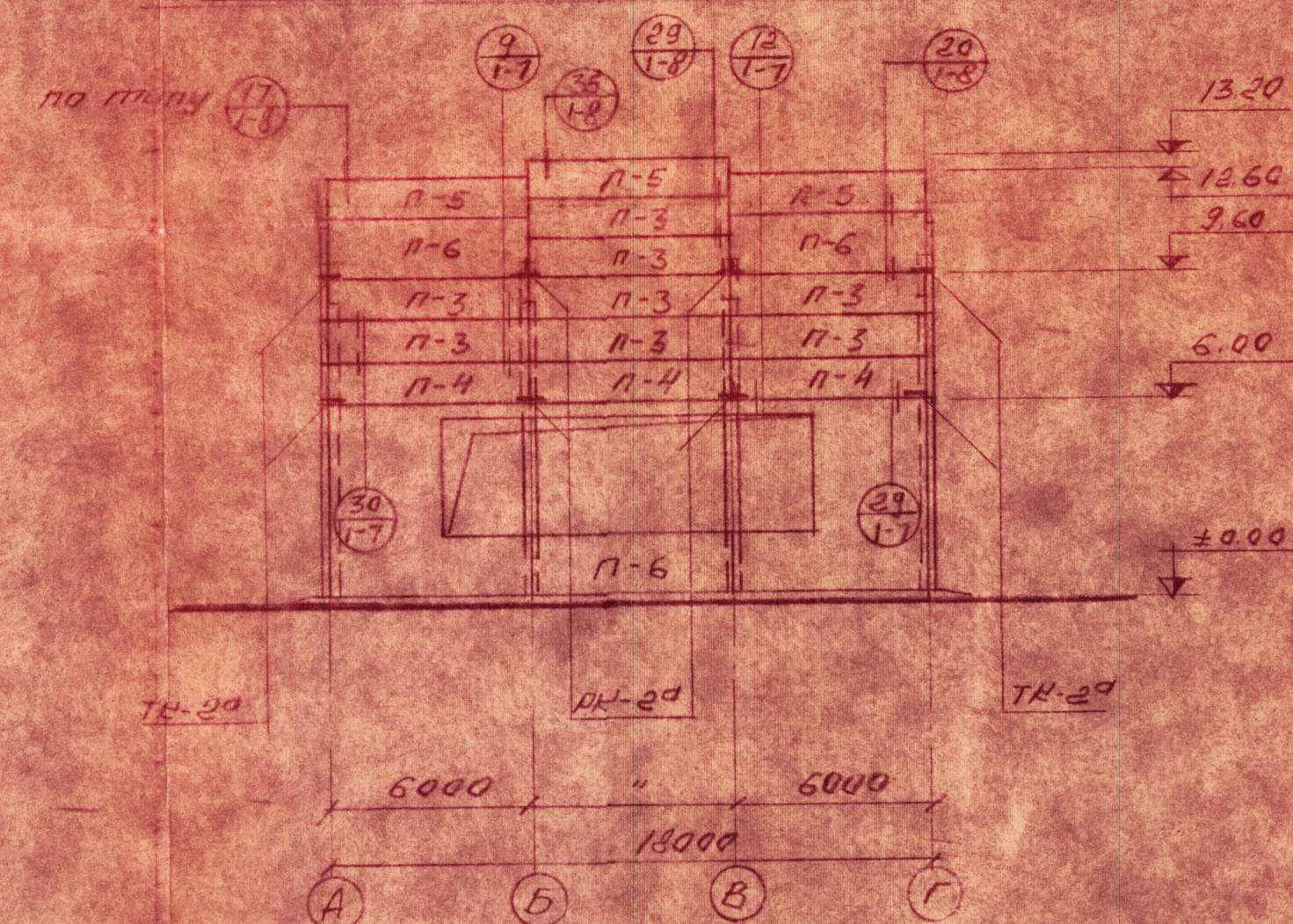
МОНТАЖНАЯ СХЕМА СТЕНОВЫХ ПАНЕЛЕЙ ПО ОСИ 8
