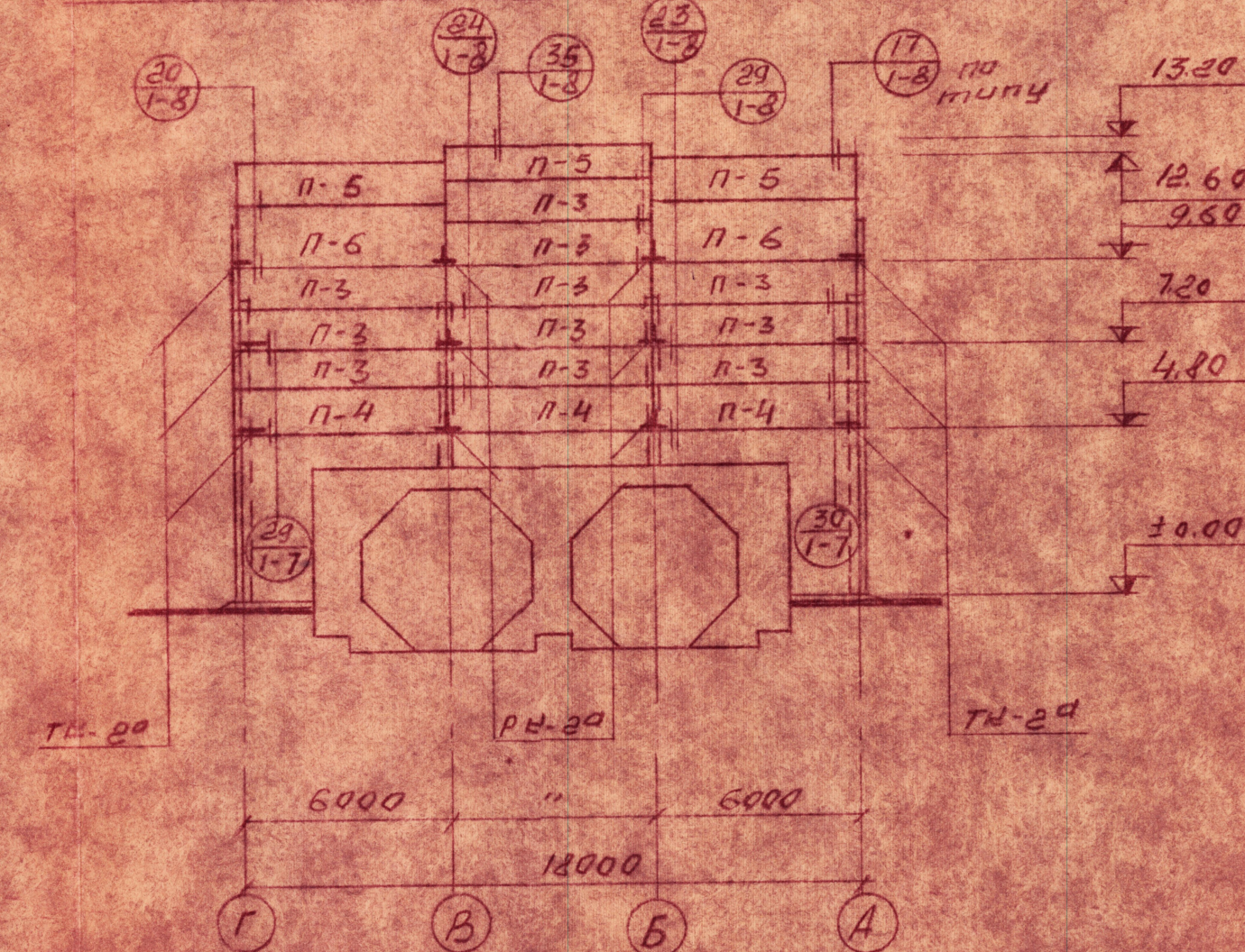
МОНТАЖНАЯ СХЕМА СТЕПОВЫХ ПАНЕЛЕЙ ПО ОСИ "I"
